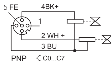
输出信号连接器 M12
