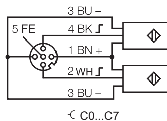
输出信号连接器 M12
