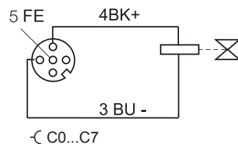
输出信号连接器 M12
