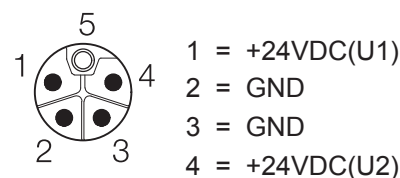
POWER AUX M12接口
