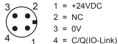
IO-Link M12接口
