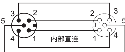
IO-Link M12接口 扩展 M12接口
