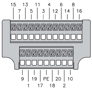
弹片夹紧式接线端子 引脚分配
