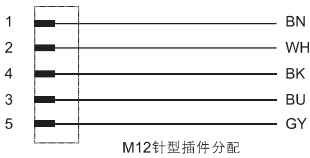
M12针型插件分配
