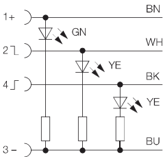
带3个LED灯，适用于PNP传感器
